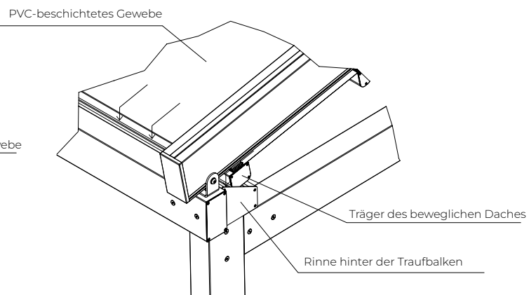
Detail Nr. 4
