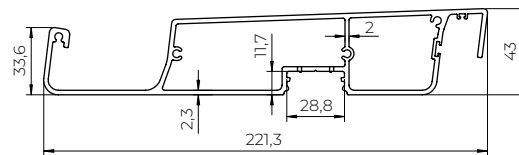
Querschnitt des Lamellenprofils mit LED-Nut (221x43)
