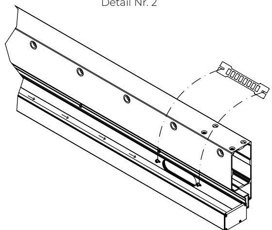
Detail Nr. 2
