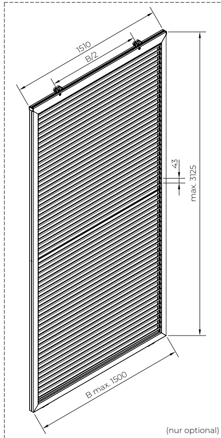
Optional - Rahmen mit Federn im Abstand von 43 mm
