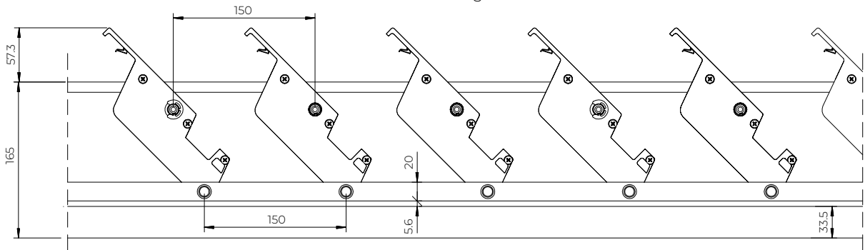
Lamellen geöffnet 45°
