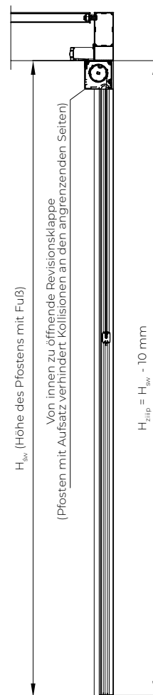
Vertikalschnitt ZiiiP in der Pergola SB400
