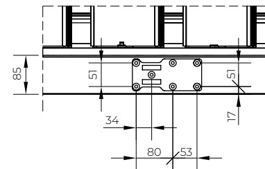
Motorbefestigung
