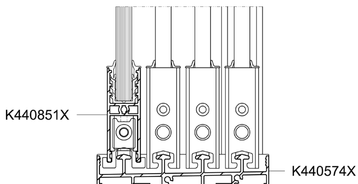
Schiebetüren fünf- blättrig / zehnblättrig
