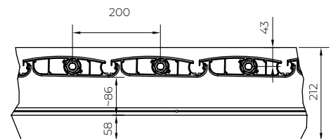
Geschlossene Lamellen
