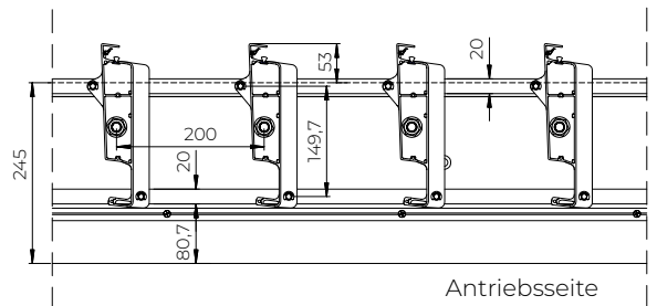
Lamellen geöffnet 90°
