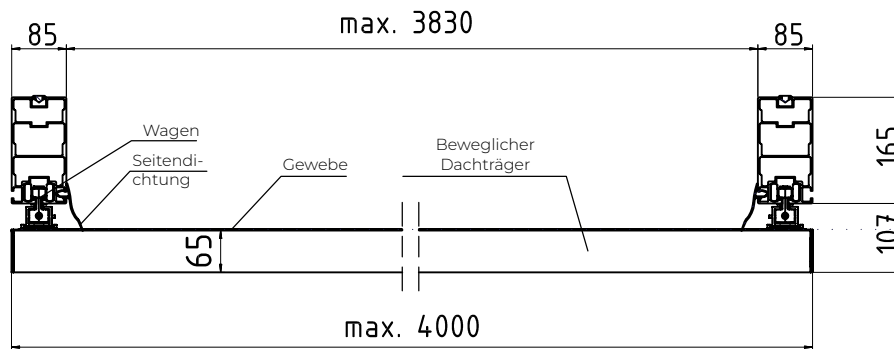
Querschnitt des Daches (Einzelversion)
