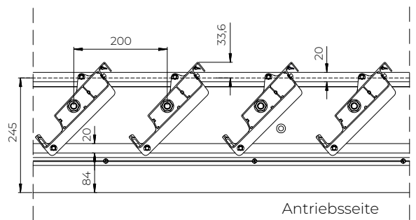
Lamellen geöffnet 45°
