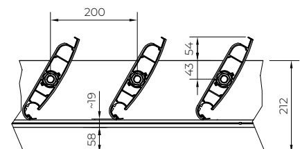
Geöffnet
