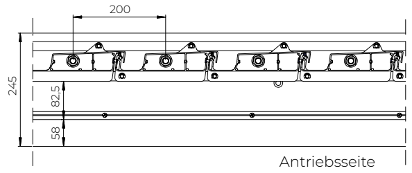
Geschlossene Lamellen
