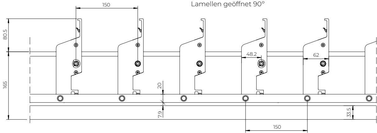
Lamellen geöffnet 90°
